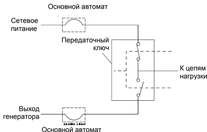
Рисунок 2.1. Основная резервная электрическая система
