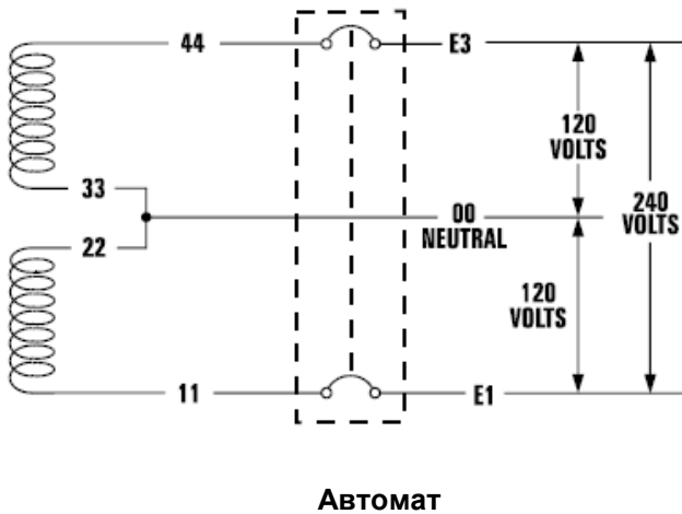
Рисунок 1.2. Статор 4 вывода, 1 фаза
