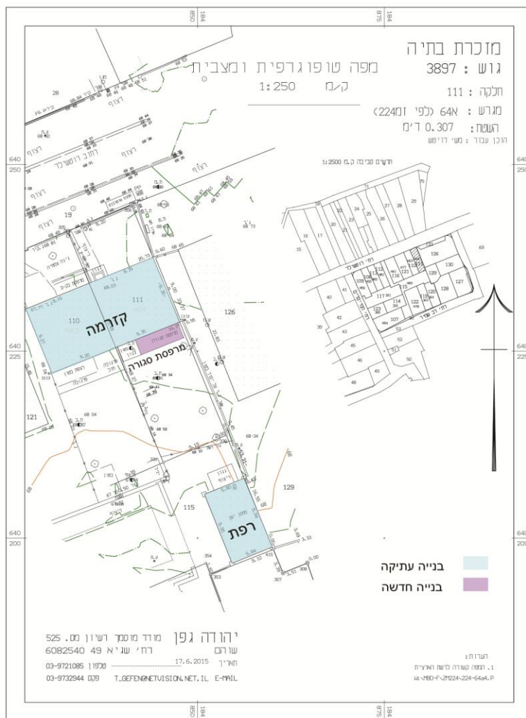
30. תוכנית טופוגרפית (ערך: י' גפן, 2015)
