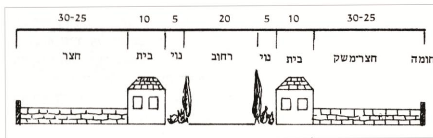
5. חתך סכמטי של רחוב במושבה עברית (מתוך: בן ארצי, 1988)
