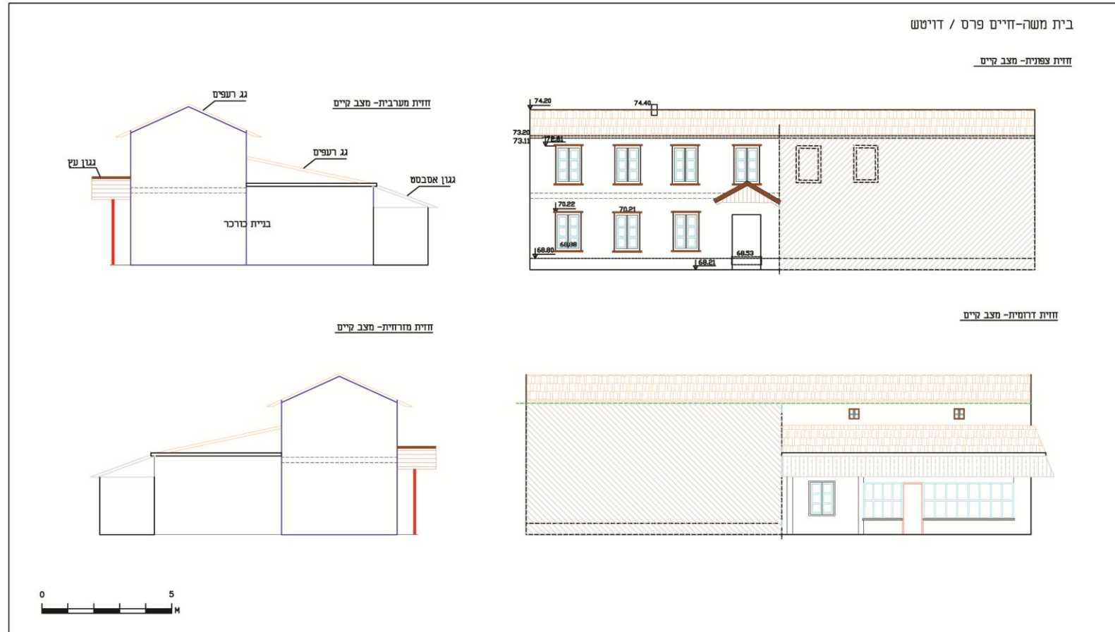
44. חזיתות מצב קיים (ערכה: מסיקה 2015)
