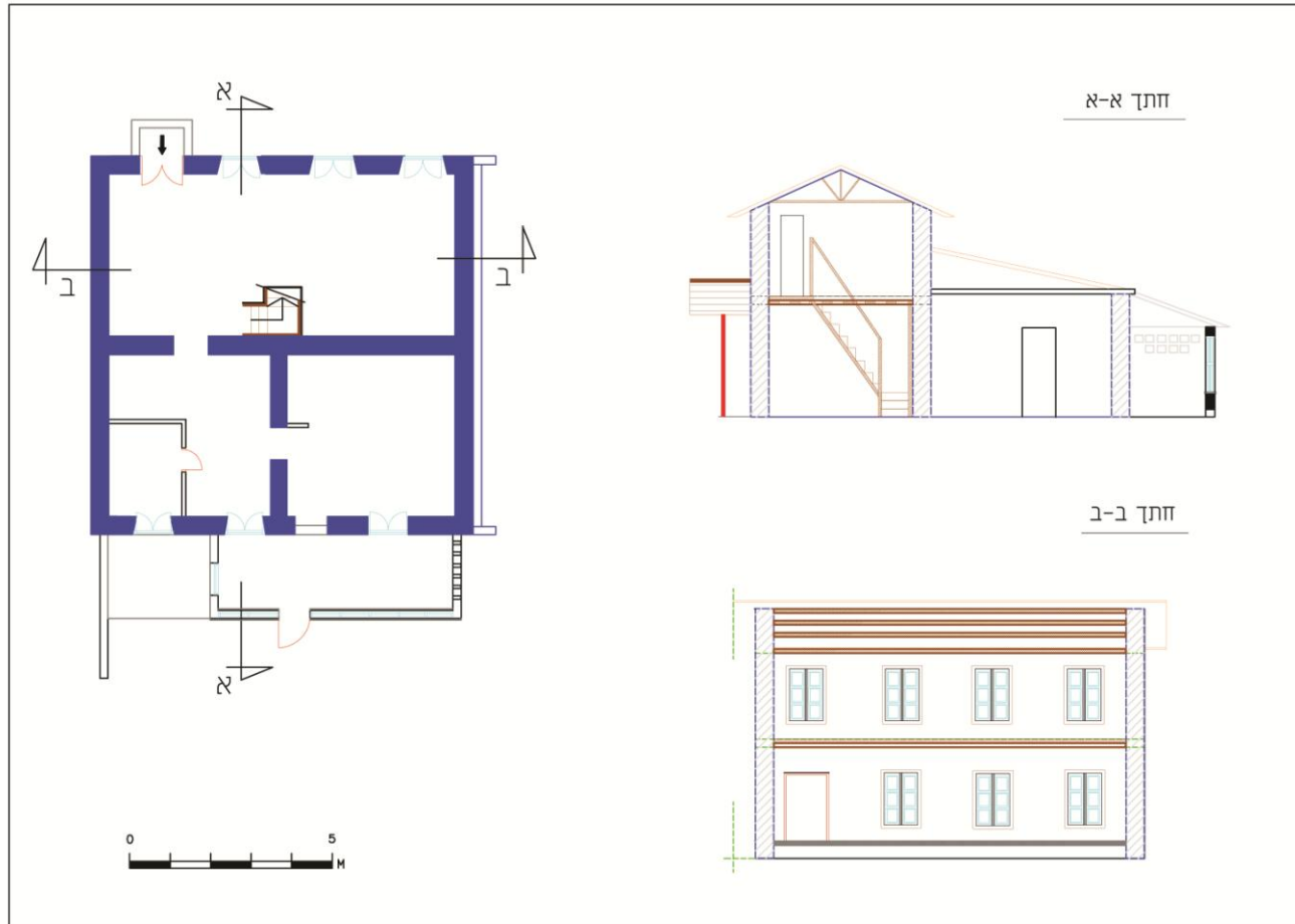
43. חתכים מצב קיים (ערכה: מסיקה 2015)
